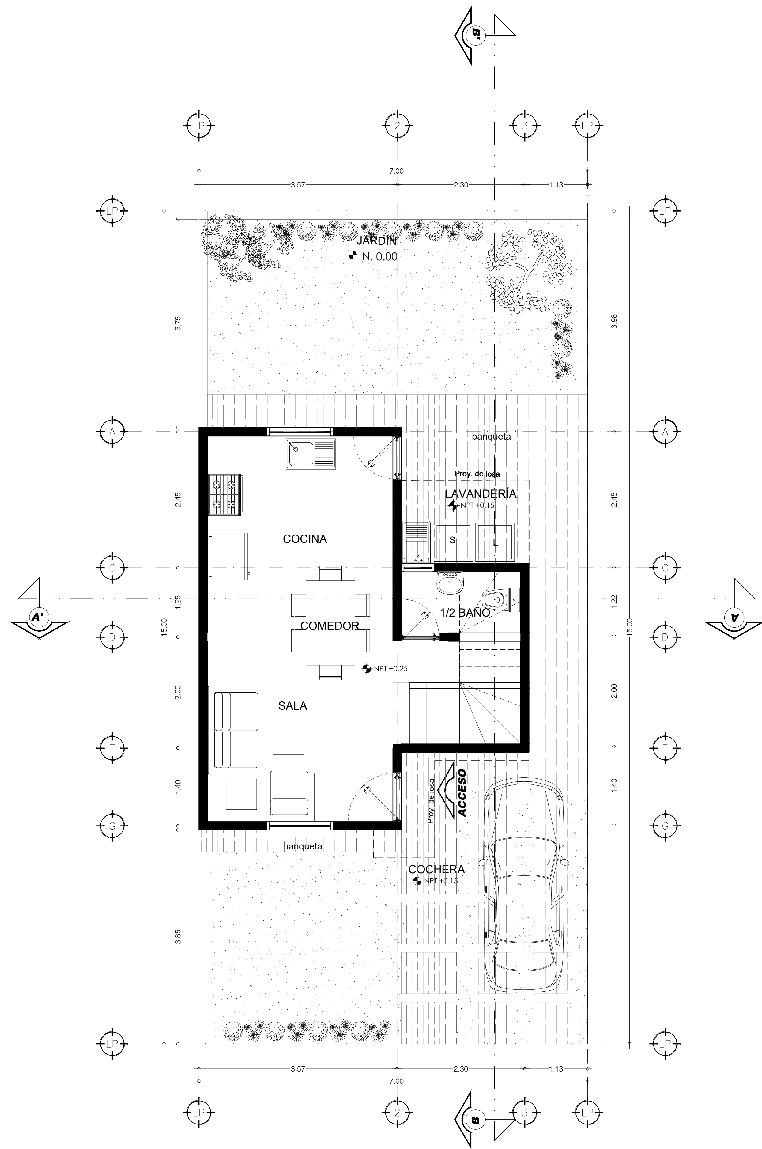
PLANTA BAJA
